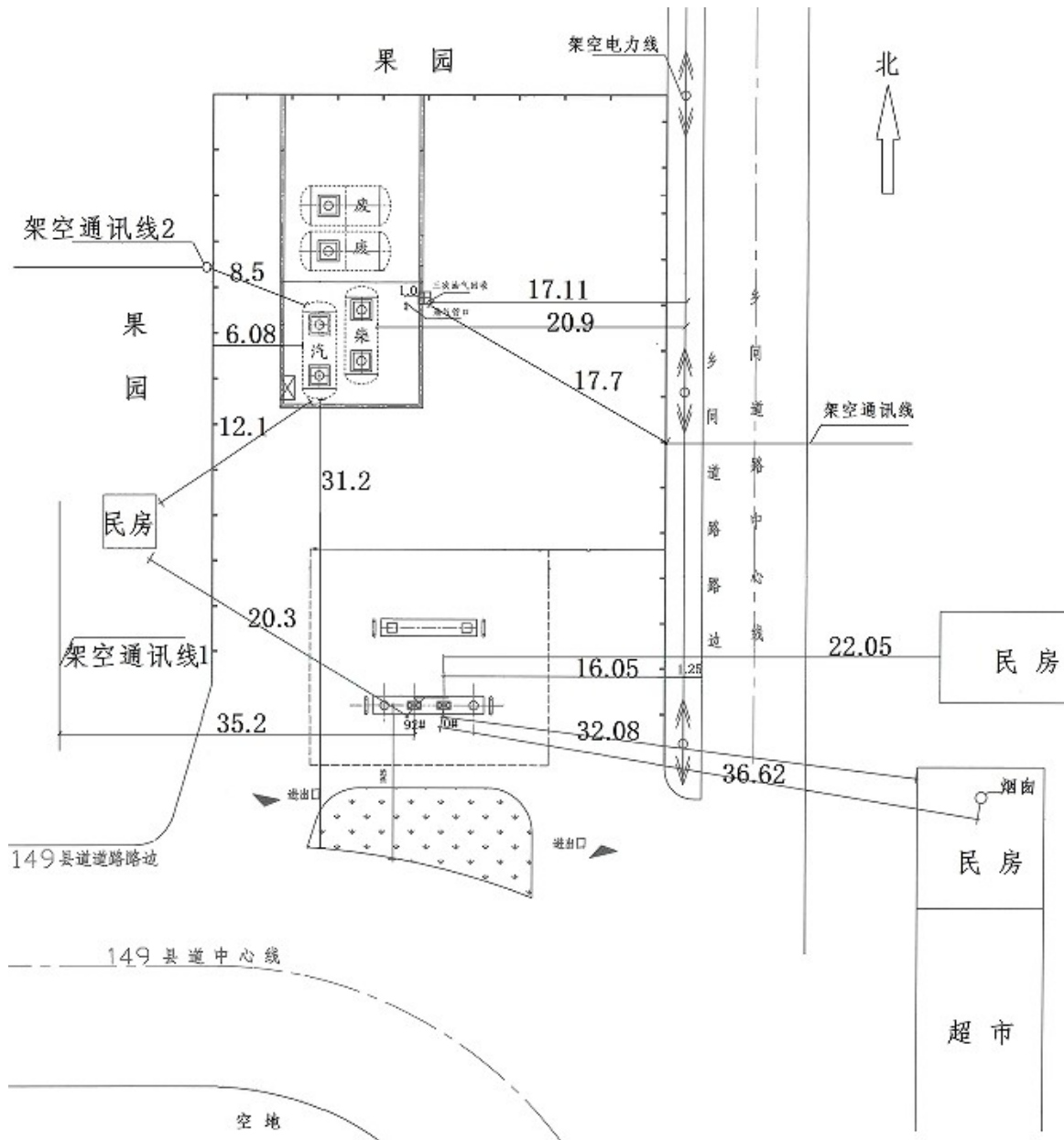
图 2.4-1 周边环境图
