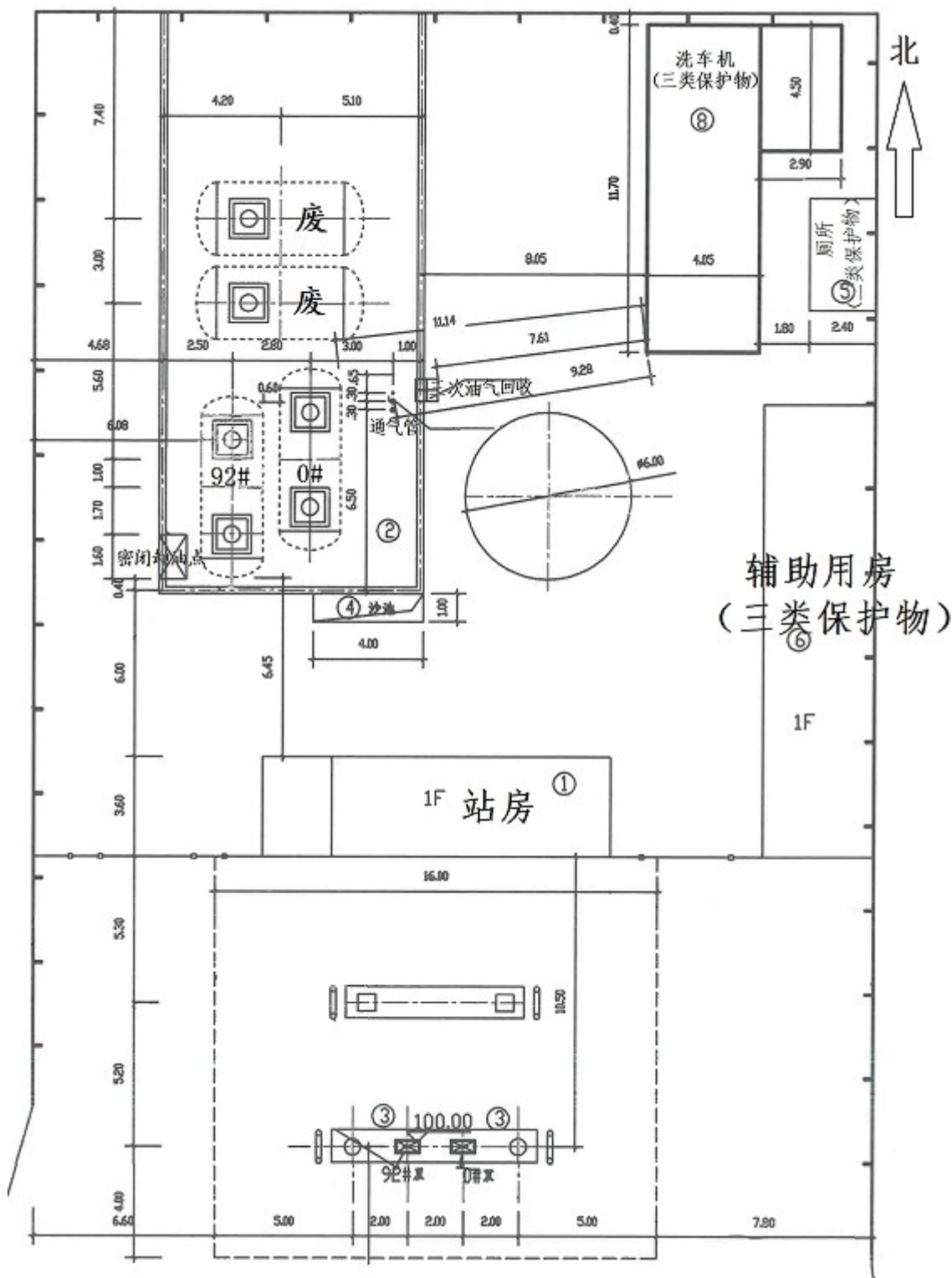
图 2.5-1 平面布置图
