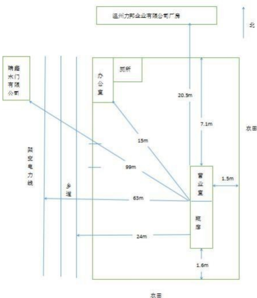
图 2.2-2 周边环境及总平面布置图
