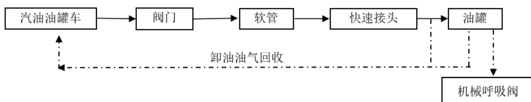
图 2-2 汽油卸油及卸油油气回收工艺流程简图
