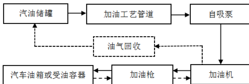
图2-4 汽油加油工艺流程简图
